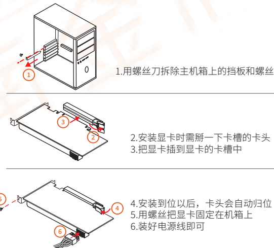
图2-10 显卡安装
