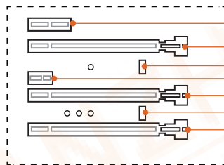
图2-4 PCI扩展插槽
